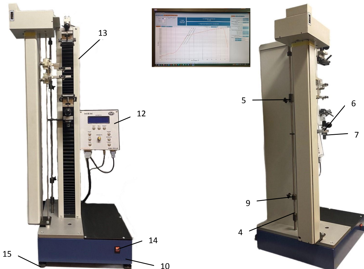
Мал.1 – Загальні вузли (вигляд спереду)
